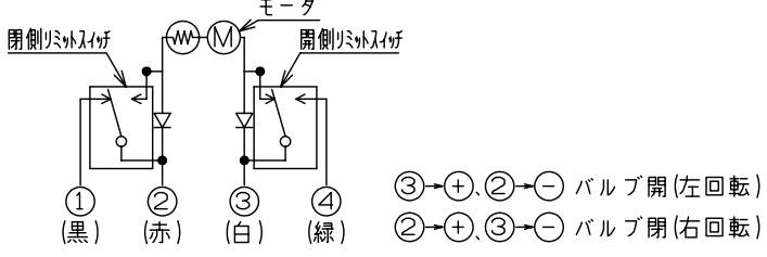
回路図 ※全閉状態を示す。
